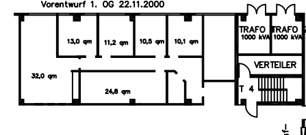
Bestand 12.03.2002 C:\DWG\BUERO\R400-6.dwg Vorentwurf 1. OG 22.11.2000
